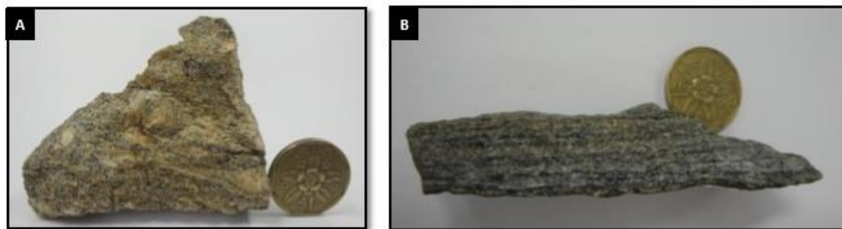
Figura 3: Amostras macroscópicas dos charnockitos da Suíte Córrego Fortaleza. Em (A) observa-se uma amostra com porfiroblastos de cor rosa claro (k-feldspato) e em (B) observa-se o bandamento.
