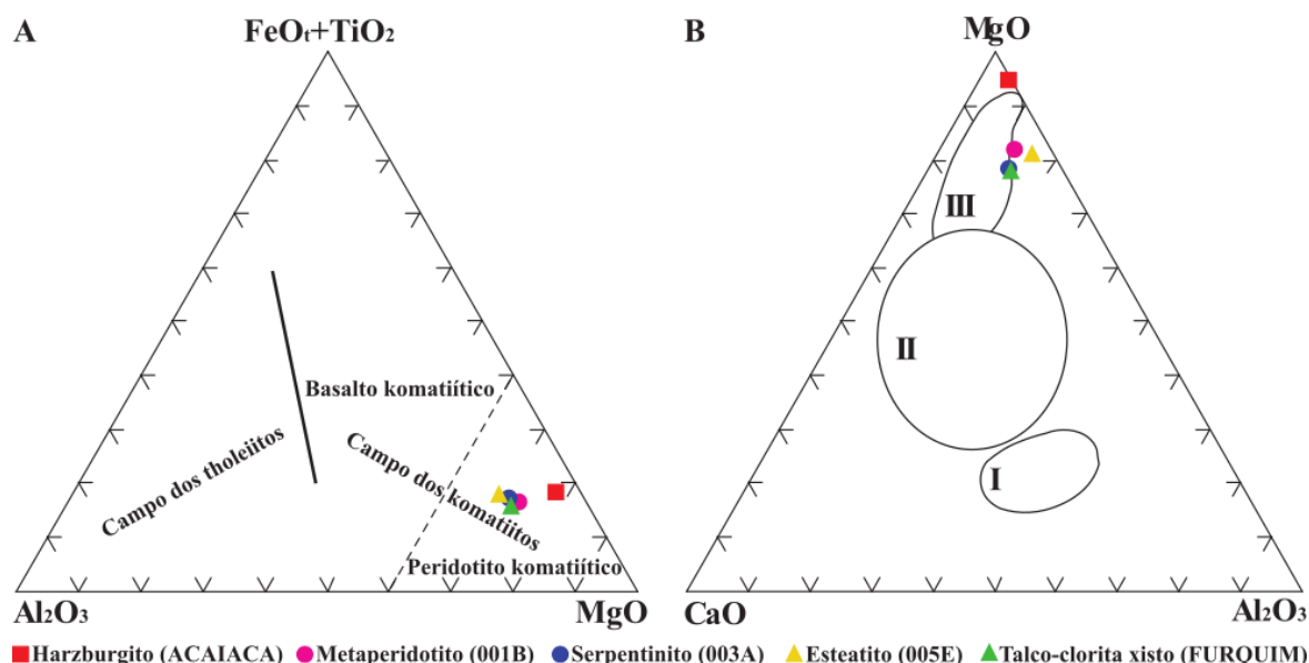
Figura 8. Diagramas ternários. A – diagrama AFM [ \text{Al}_2\text{O}_3 -( \text{FeO}+\text{TiO}_2 )- \text{MgO} ] de Jensen(1976)para classificação de rochas ultramáficas. B - diagrama ternário \text{MgO} - \text{CaO} - \text{Al}_2\text{O}_3 para komatiitos e rochas afins de Barberton, adaptado de Vilijoen et al. (1982), onde: I - Basaltos tholeiíticos; II - Basaltos komatiíticos e III - Peridotitos komatiíticos.
