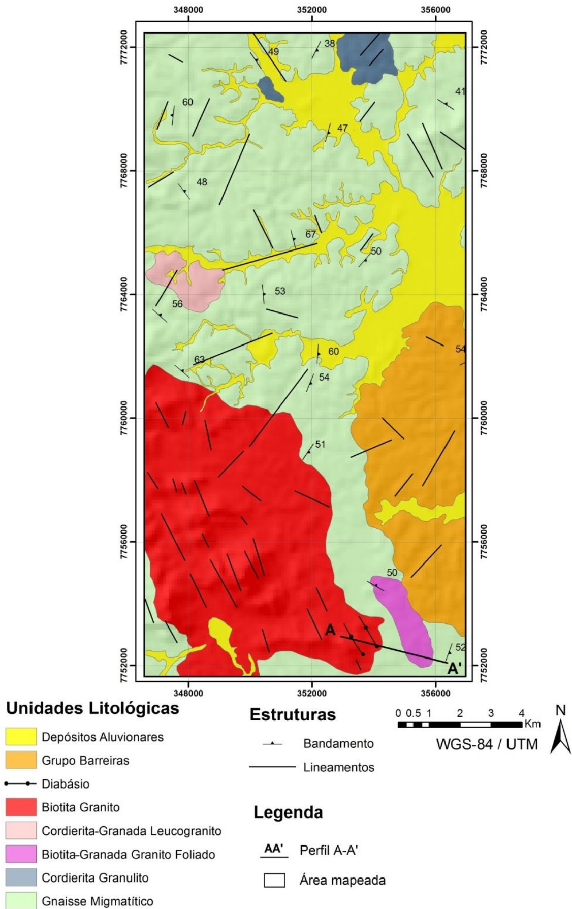
Figura 3. Mapa geológico em escala 1:50.000.
