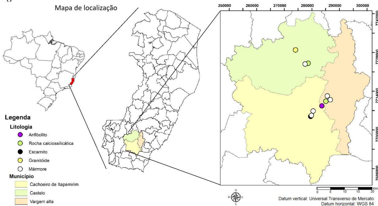
Figura 1. Localização da área estudada com a distribuição espacial dos pontos estudados.
