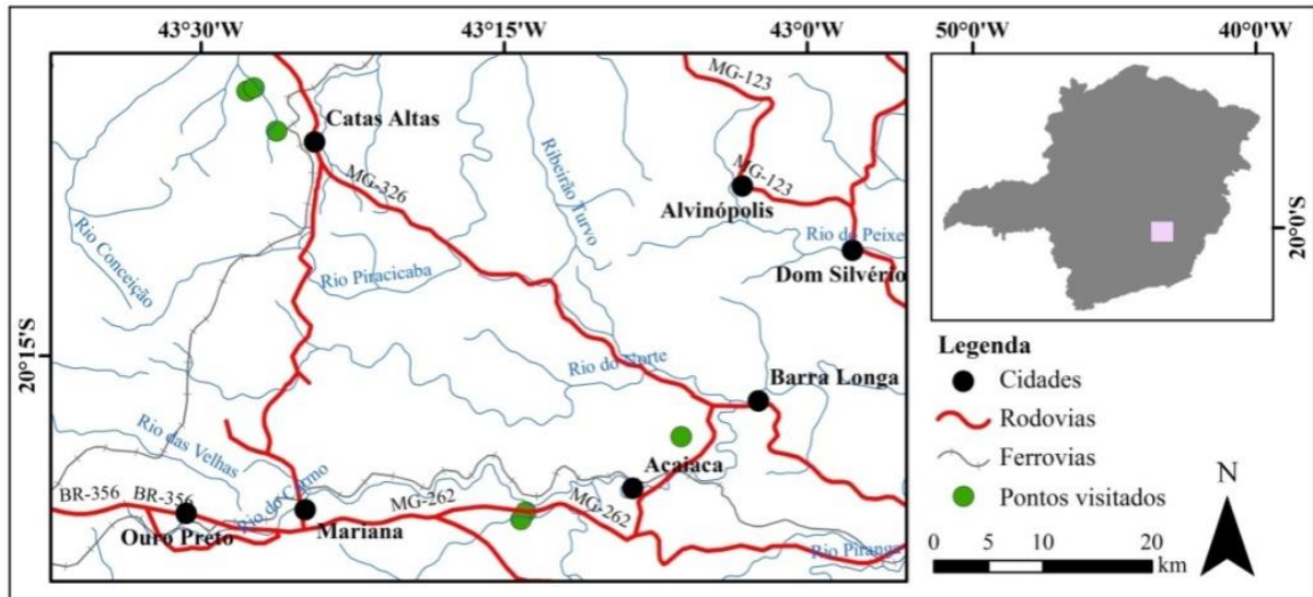
Figura 2. Localização e vias de acesso aos pontos visitados.
