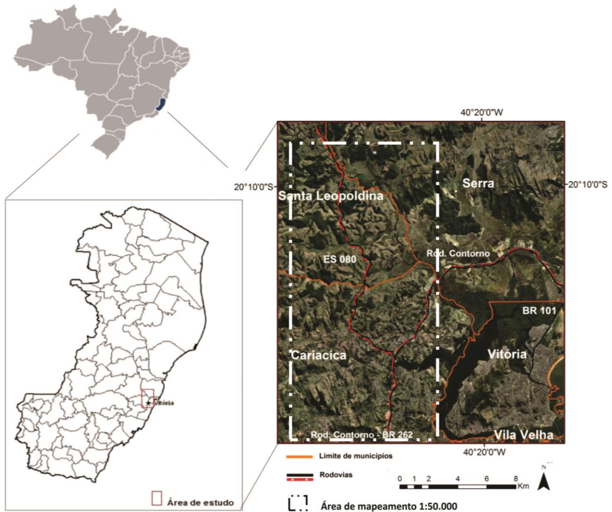
Figura 1. Mapa de localização da área de estudo, demarcada pelo polígono tracejado.
