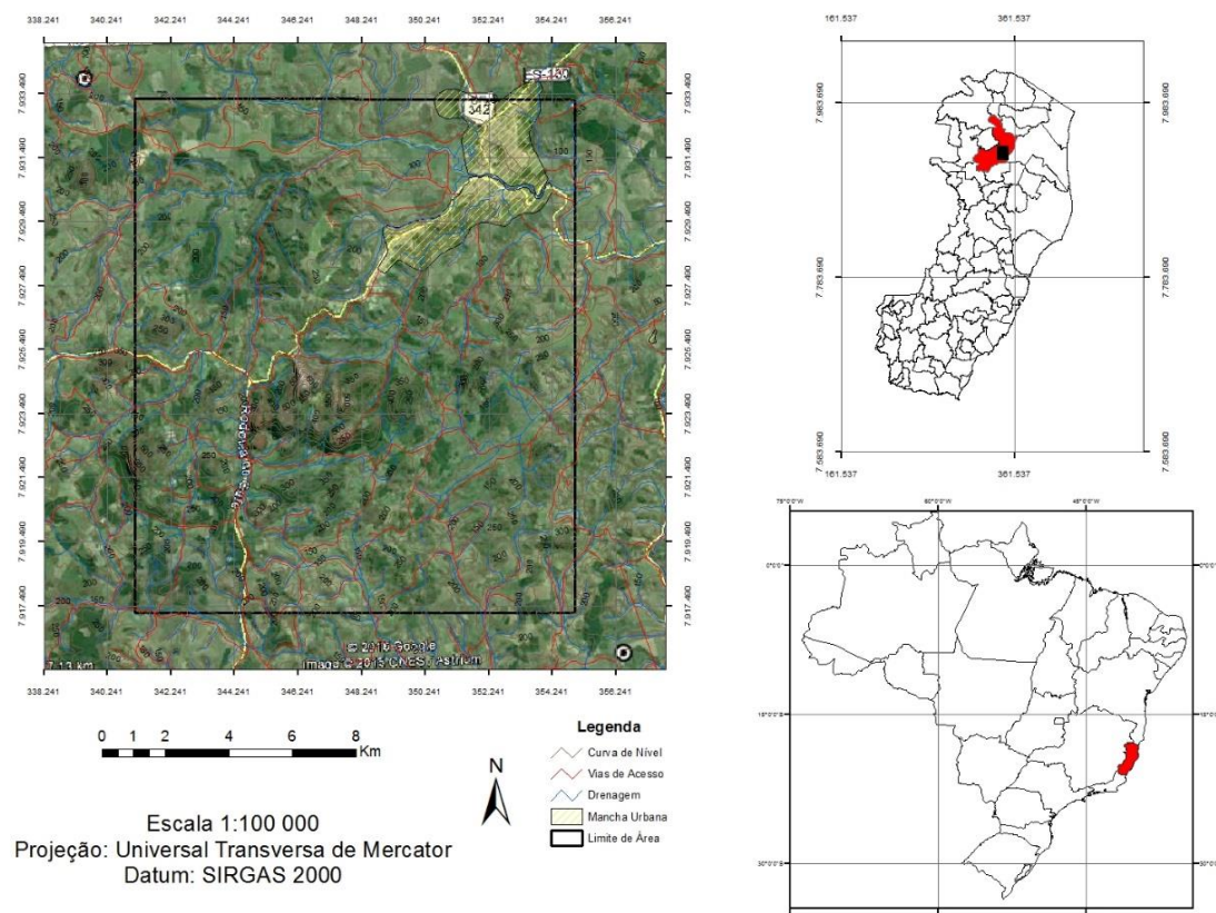
Figura 1. Mapa de localização da área, no município de Nova Venécia, Espírito Santo.
