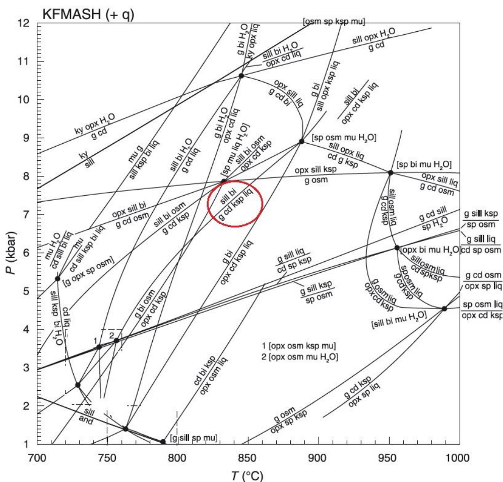
Figura 5. Grade petrogenética do sistema KFMASH estabelecendo campos de pressão e temperatura, com destaque para a reação de geração de granada e cordierita a partir de biotita e sillimanita (modificado de WHITE et al., (2007).
