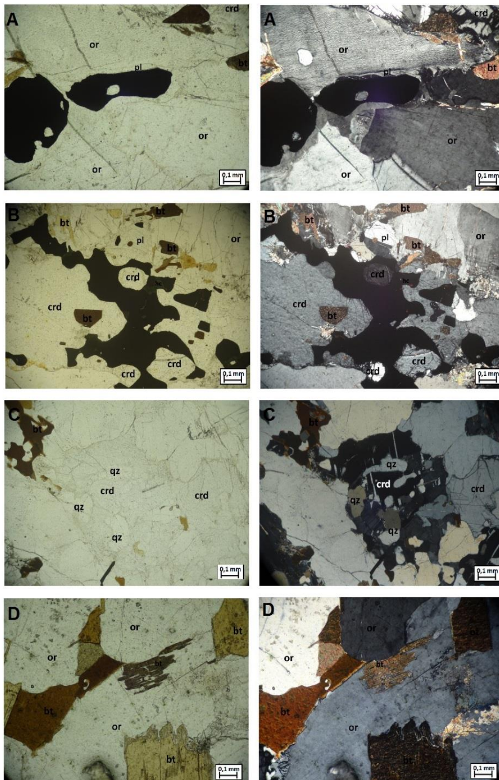
Figura 4. Fotomicrografia de cordierita granulito do Ponto 25. (A) Filme de plagioclásio envolvendo mineral opaco. (B) Mineral opaco associado à hercinita e a cordierita. (C) Cordierita com inclusões de quartzo amebóide. (D) Palheta de biotita com simplectita de quartzo. Or = ortoclásio; PL = plagioclásio; crd = cordierita; bt = biotita; qz = quartzo. As fotomicrografias das colunas a esquerda são em polarizada paralela e as fotomicrografias a direita são em luz polarizada cruzada.
