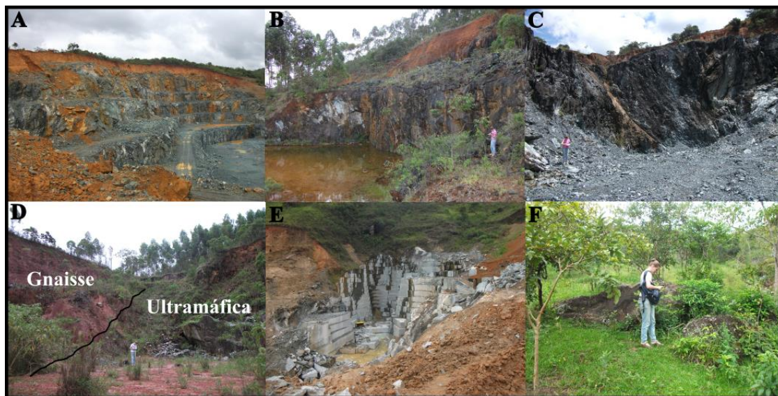
Figura 5. Fotos dos afloramentos visitados. A – Pedreira de metaperidotito (Ponto 001). B e C – Pedreira desativada de serpentinito (Ponto 002 e 003). D – Pedreira desativada de talco xisto, onde se observa o contato da rocha metaultramáfica com o gnaiss (Ponto 004). E – Pedreira de esteatito (Ponto 005). F – Blocos de harzburgito (Ponto 006).
