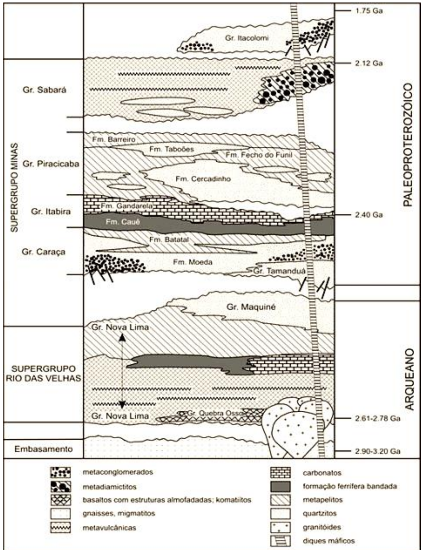
Figura 4. Coluna estratigráfica do Quadrilátero Ferrífero retirada de Alkmim e Marshak (1998).
