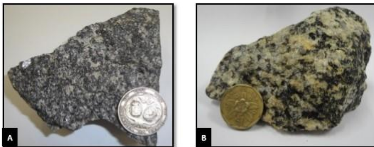
Figura 2: Amostras do charnockito da Suíte Monte Verde. Em (A) rocha maciça de coloração cinza e em (B) rocha ligeiramente alterada de coloração esbranquiçada.
