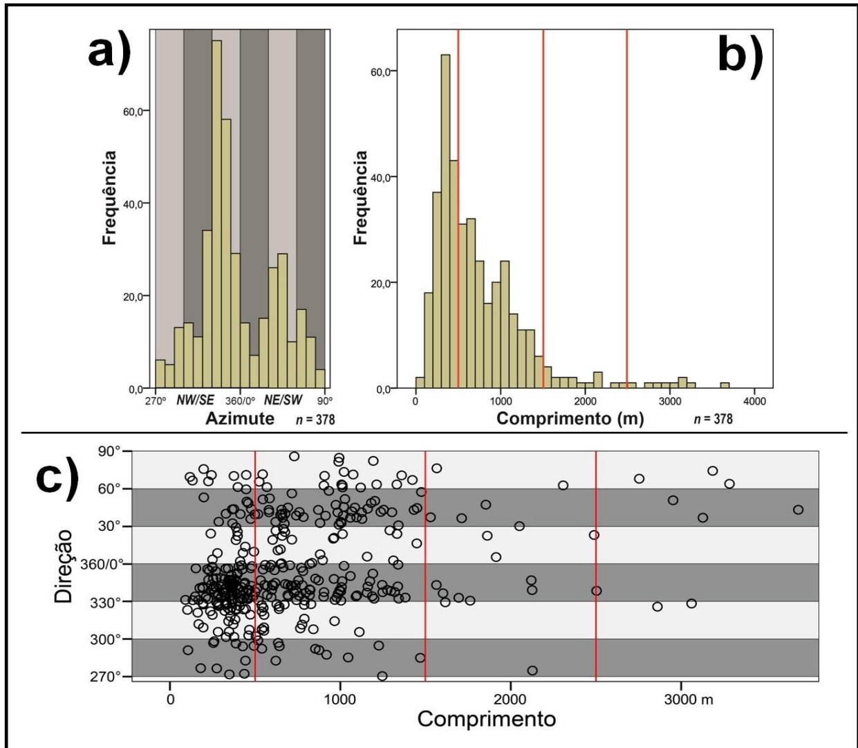
Figura 7. Histograma de comprimento e direção e gráfico de direção versus comprimento dos lineamentos extraídos por fotointerpretação. Em a) é mostrado o histograma de direção; em b) o histograma de comprimento; e em c) o gráfico de direção versus comprimento (n:378).
