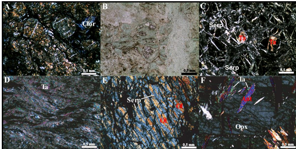
Figura 6. Fotomicrografias. A – Metaperidotito com textura blaschumilática e grãos de clorita (Clor). B – Metaperidotito com textura blaschumilática e seção basal octaédrica de piroxênio. C – Serpentinito com serpentina (Serp) e talco (Ta). D – Esteatito com textura lepidoblástica dada por talco (Ta). E – Serpentina (Serp) preenchendo fraturas em grão de olivina (Ol). F – Antofilita (Ant) incluída em ortopiroxênio (Opx) com suas bordas substituídas por talco (Ta).
