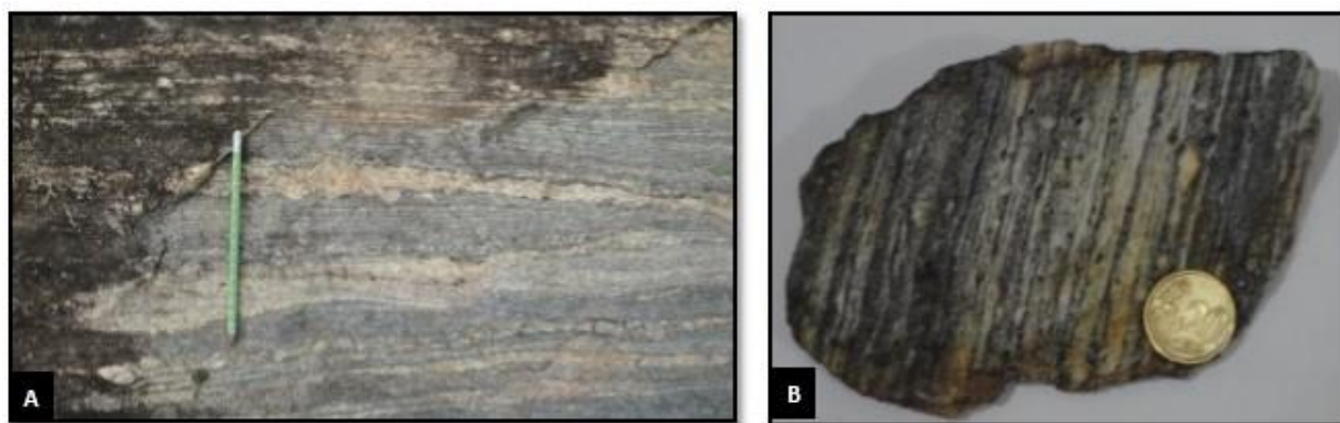
Figura 6: Em (A) afloramento evidenciando o bandamento gnáissico do e em (B) amostra de mão do Leucogranitogneissificada da Suíte São João do Paraíso.
