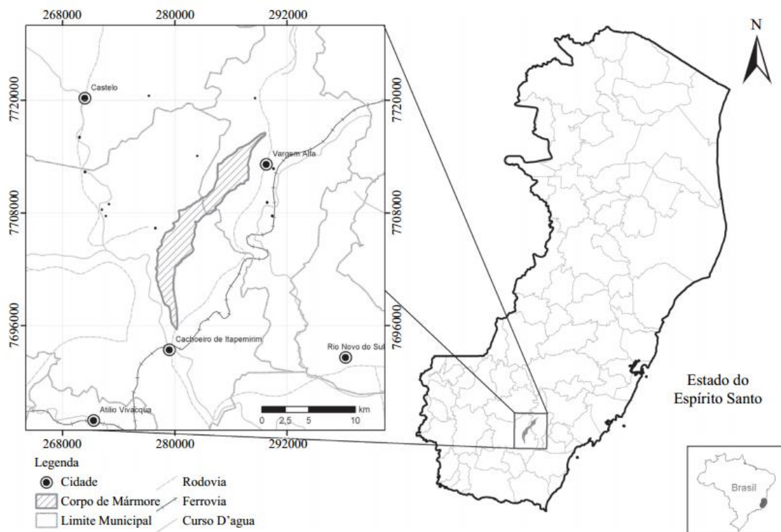
Figura 2. Lente de mármore do Complexo Paraíba do Sul.
