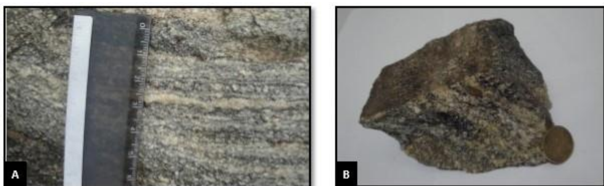
Figura 4: Amostras macroscópicas do Biotita-Gnaiss-Milonítico. Em (A) e (B) observa-se porfiroclastos de plagioclásio.
