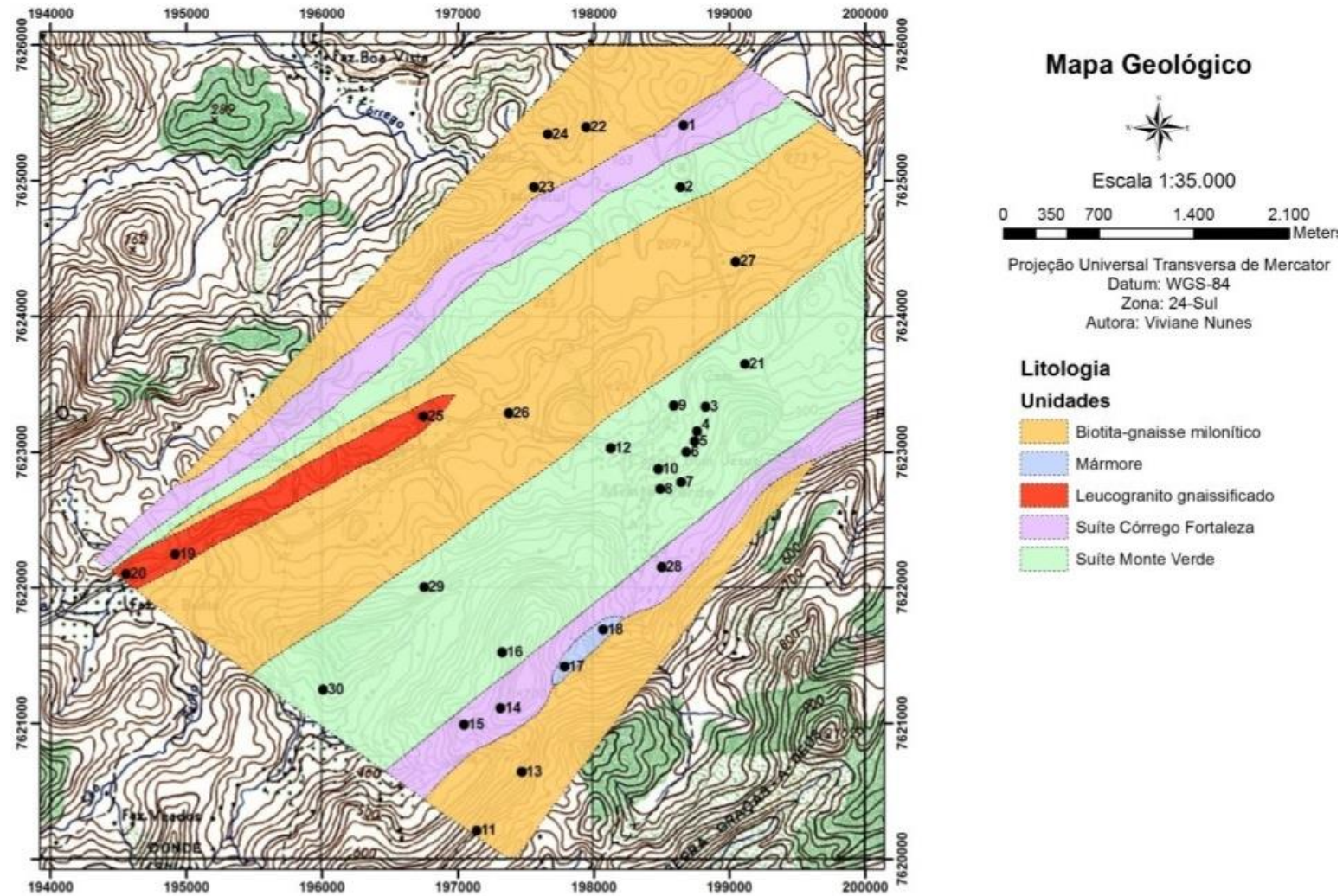
Figura 1. Mapa Geológico da região de Monte Verde-RJ na escala 1:35.000
