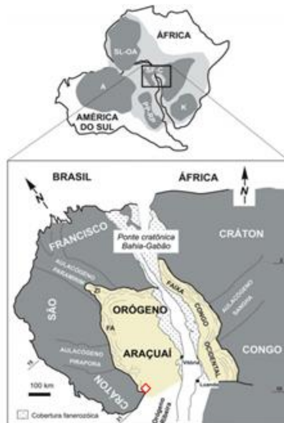
Figura 3. O Orógeno Araçuai na região central do Paleocntinente Gondwana. O retângulo vermelho indica localização da região estudada (adaptado de ALKMIM et al., 2006).
