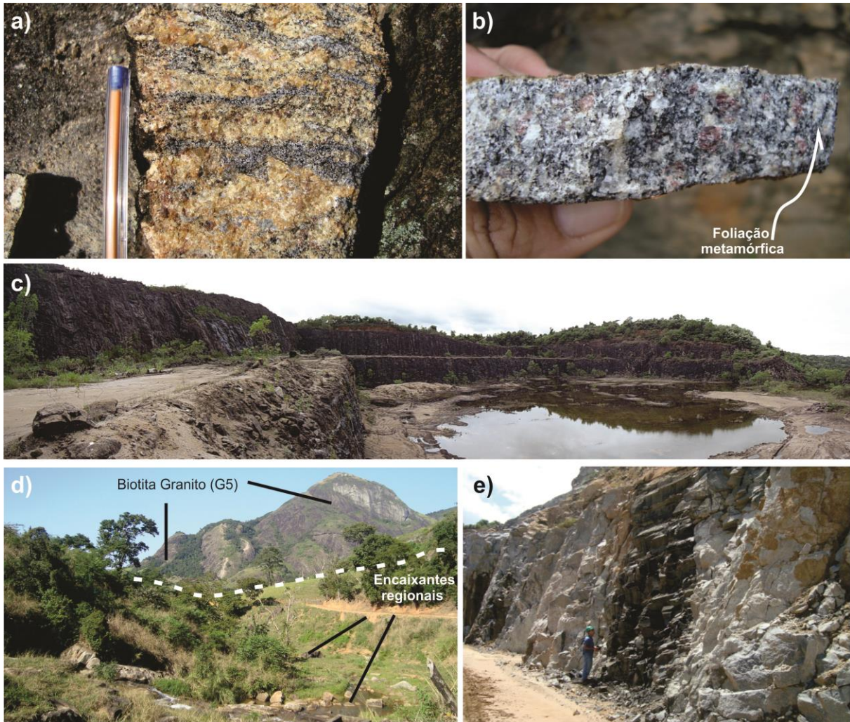
Figura 5. Aspectos de campo da área de estudo. a) Amostra de gnaiss migmatítico; b) amostra de biotita-granada granito foliado; c) afloramento de cordierita granulito; d) contraste geomorfológico entre as rochas do biotita-granito e suas encaixantes (gnaiss migmatítico); e) dique de diabásio intrudindo biotita-granito.
