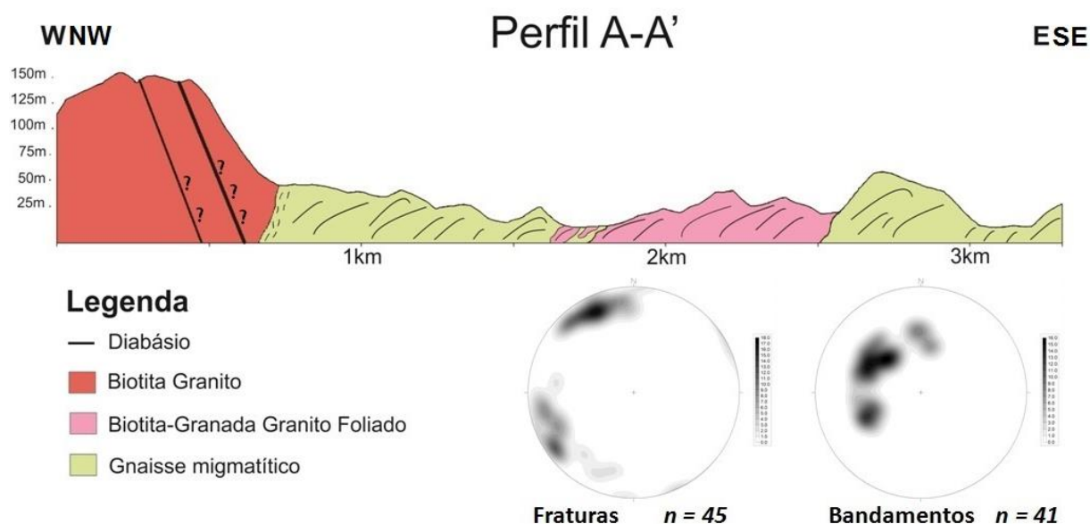
Figura 4. Seção geológica A-A' construída em escala 1:50.000.
