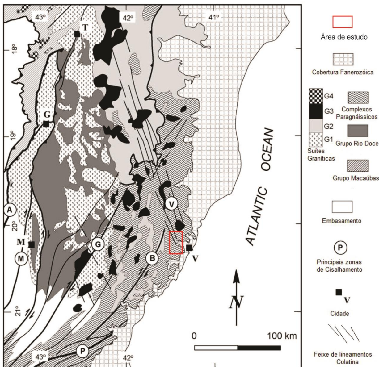
Figura 2. Mapa geológico do Orógeno Araçuaí, com destaque para a área de estudo, demarcada em vermelho. Zonas de Cisalhamento: A: Abre Campo; M: Manhuaçu; G: Guaçuí; B: Batatal; P: Além Paraíba. Cidades: V: Vitória, G: Governador Valadares, T: Teófilo Otoni (ALKMIN et al., 2006).
