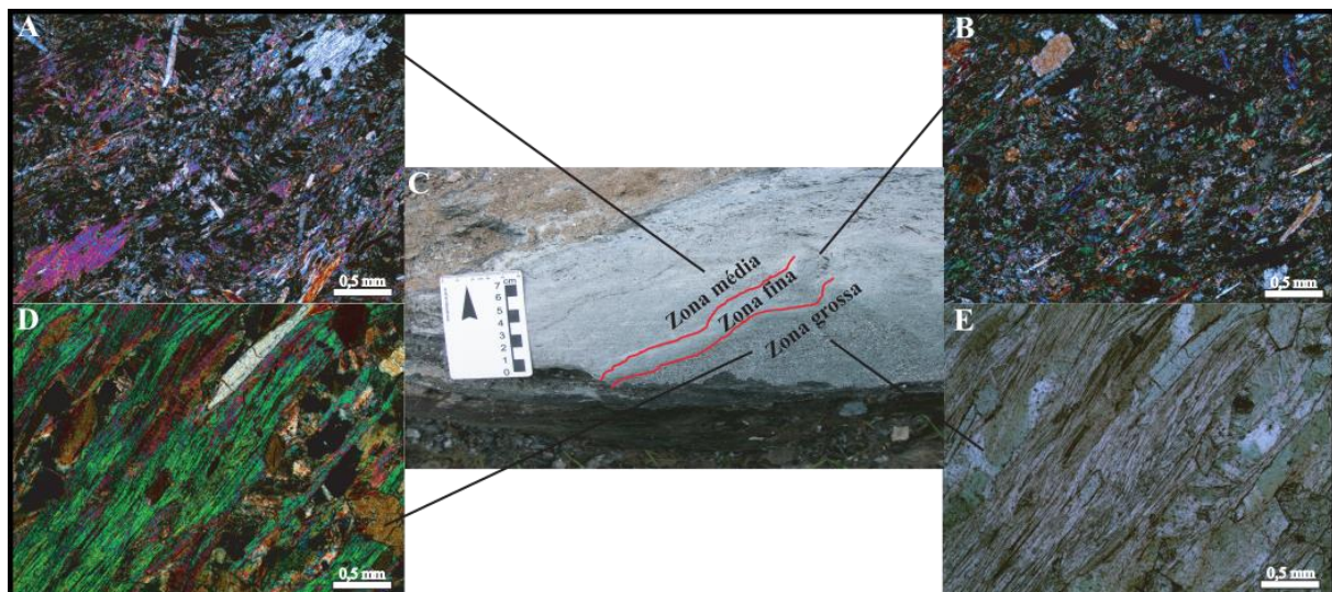
Figura 7. Zonas do black wall . A – Zona de granulação média com tremolita (Trem), clorita (Clor) e Biotita (Bt). B – Zona de granulação fina com tremolita (Trem) e talco (Ta). C – Afloramento do black wall . D – Zona de granulação grossa com tremolita (Trem), biotita (Bt) e talco (Ta), à nicóis cruzados. E – Zona de granulação grossa com tremolita (Trem), biotita (Bt) e talco (Ta), à nicóis descruzados.
