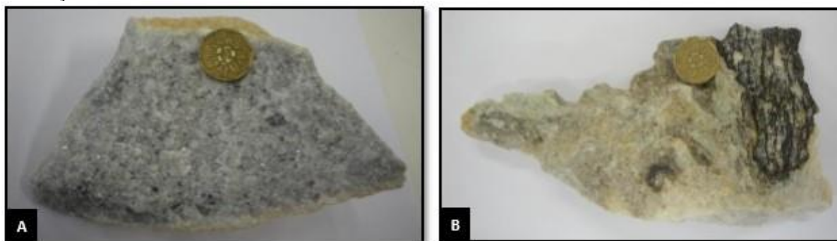
Figura 5: Amostras amacrocópicas dos mármore que ocorrem na Região de Monte Verde-RJ. Em (A), mármore cinza azulada de granulação média. Em (B), mármore branco com porções escarnitizada (verde).
